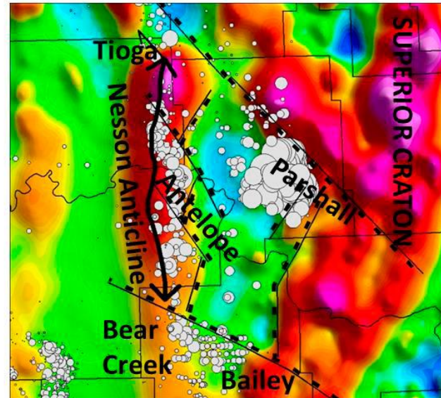
(d) Interpretation on Magnetic anomaly data
